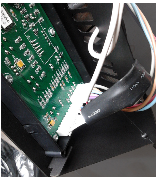
3. Connectez les faisceaux de câblage installés en usine au panneau de commande, comme illustré.
