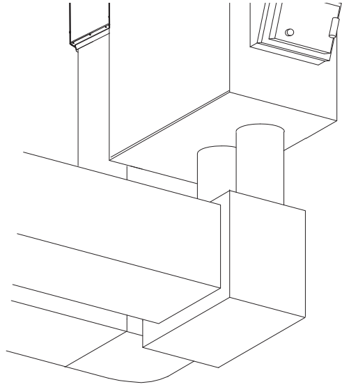
Taille de la sortie du réseau de gaines de l'air soufflé (air chaud)
