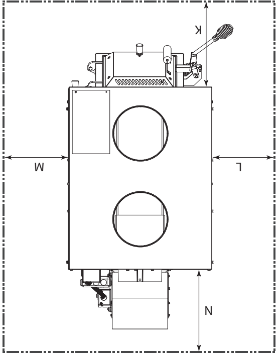
Dégagements Par Rapport Aux Matériaux Inflammables
